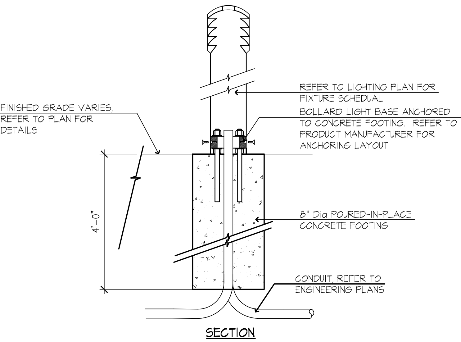
1 BOLLARD LIGHT SCALE: N.T.S
