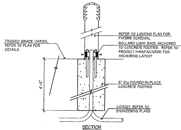
1 BOLLARD LIGHT SCALE: N.T.S.
