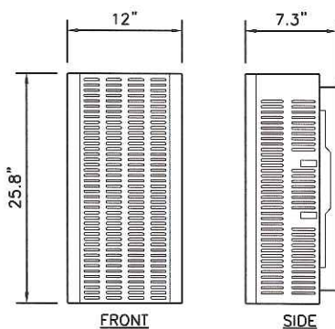
⑤ RRH SPEC. N.T.S.
