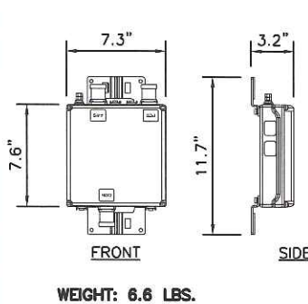
④ DIPLEXER SPEC. N.T.S.
