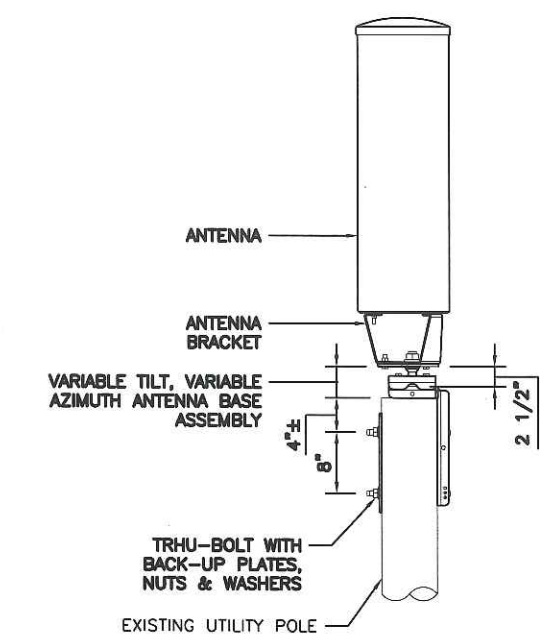
⑥ ANTENNA MOUNTING DETAIL N.T.S.
