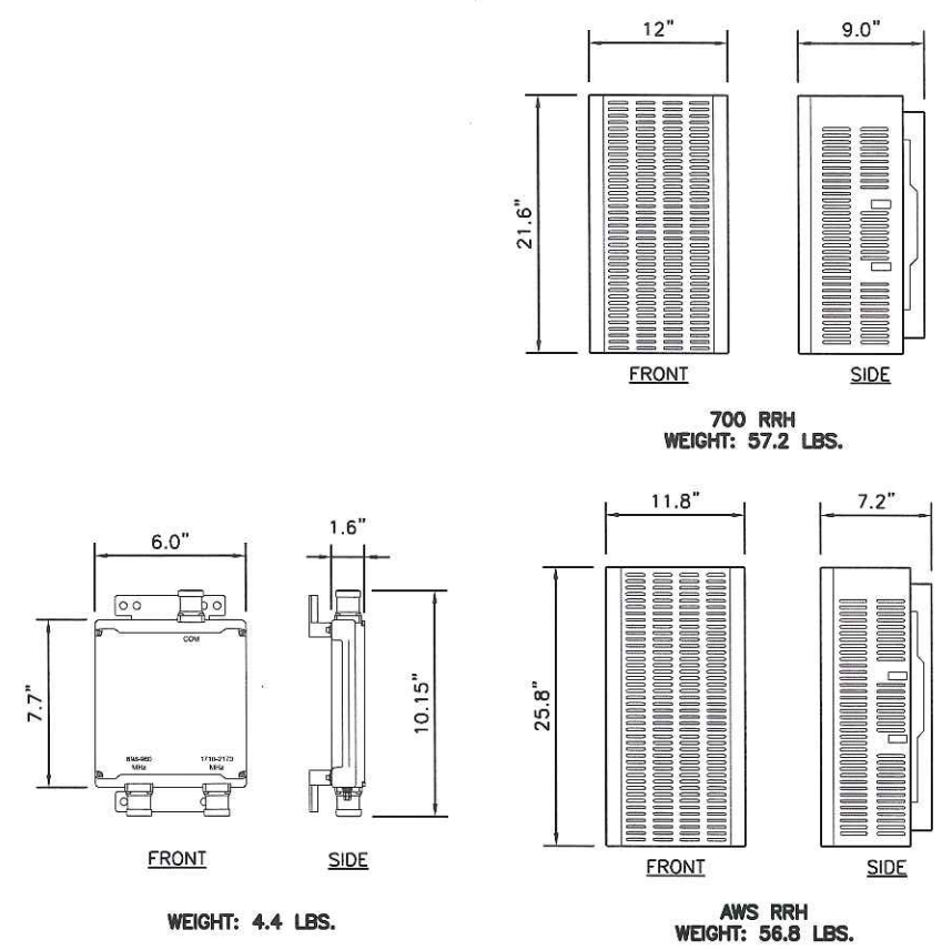
④ DIPLEXER SPEC. N.T.S.
